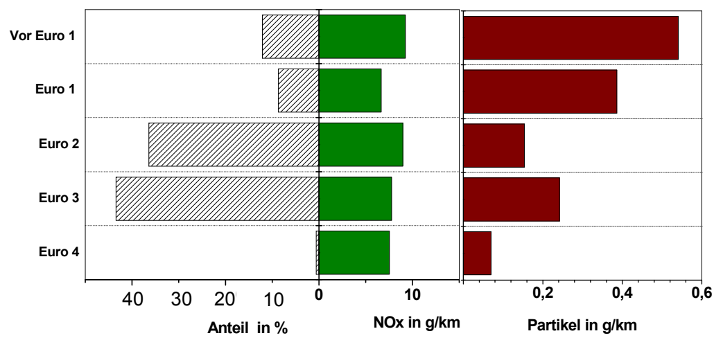
Abbildung 2-5 Schwere Nutzfahrzeuge (sNfz): Dynamische Flottenanteile und Emissionsfaktoren (Deutschland, innerorts), differenziert nach Emissionsstufen für NO x und Partikel. Bezugsjahr 2005 nach HBEFA 2.1, Mittelwert über alle sNfz [1]
