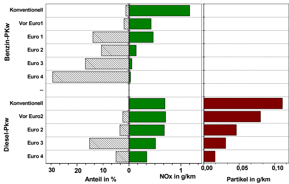
Abbildung 2-6 Benzin- und Diesel-Pkw: Dynamische Flottenanteile und Emissionsfaktoren (Deutschland, innerorts), differenziert nach Emissionsstufen für NO x und Partikel. Bezugsjahr 2005 nach HBEFA 2.1 [1]
